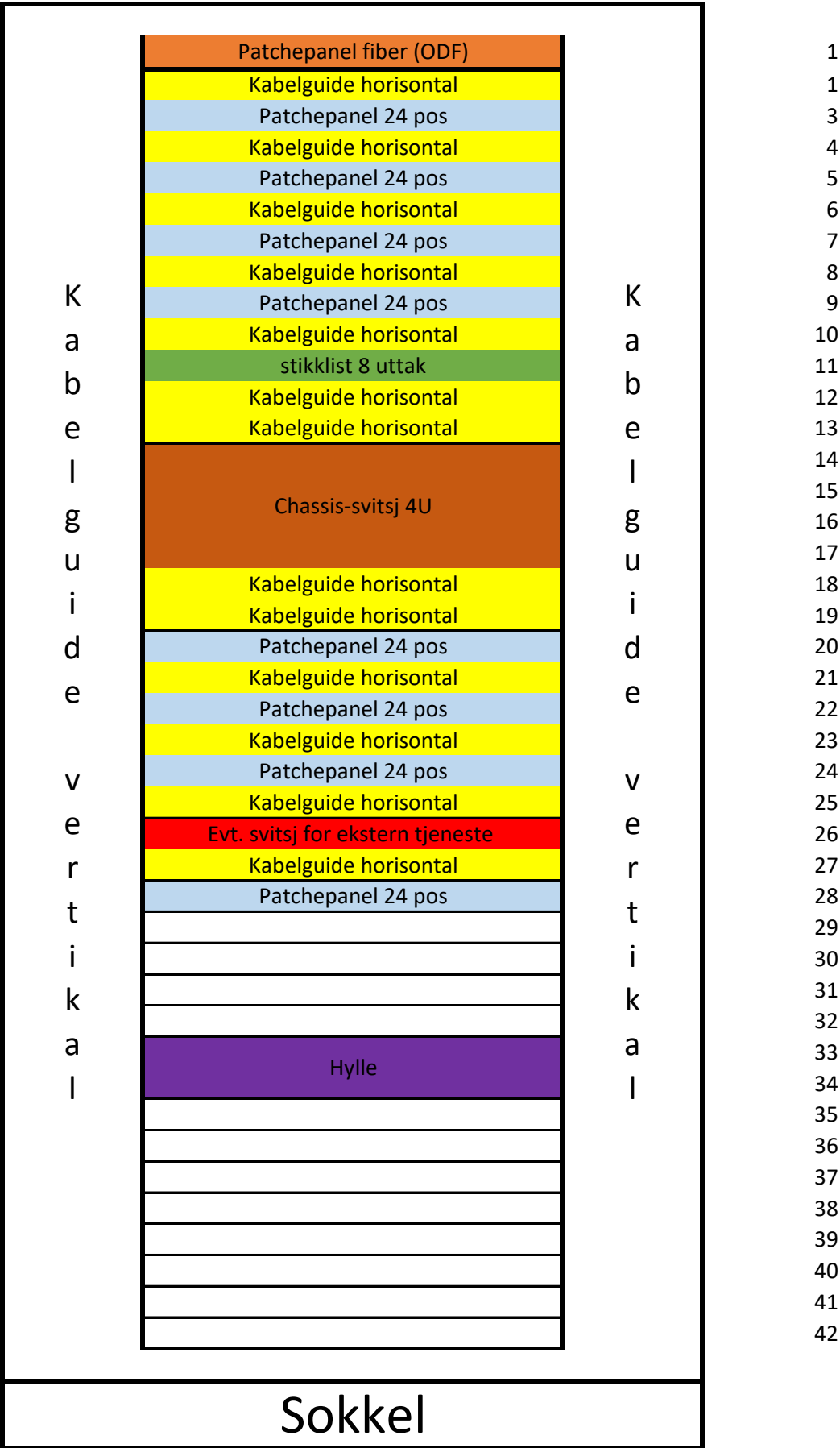
Eksempel på oppbygging av skap med 4U chassis-svitsj og TV-svitsj. Tilpasses slik at prisippet beholdes.
